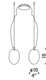
PRO•SECCO S2D 2x20W-12V G4 HSGST/UB alogeno bispina halogen bi-pin cavo elettrico 200 cm trasformatore elettronico cables length 200 cm electronic transformer
